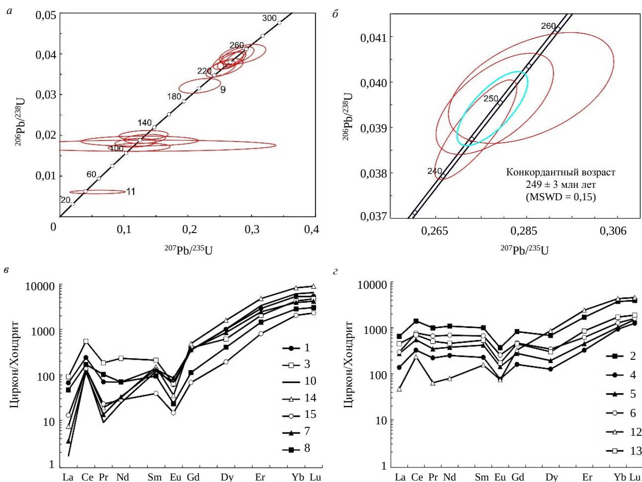
Рис.2. Диаграмма с конкордией (а, б) и спектры распределения REE (в, з), нормированные к хондриту CI, для циркона из гранитов первой фазы (обр. 2020-13) 1-15 – точки анализа
