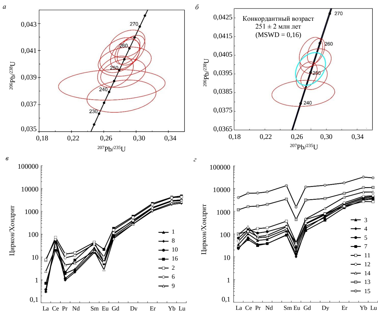
Рис.5. Диаграмма с конкордией (а, б) и спектры распределения REE (в, з), нормированные к хондриту C1, для циркона из гранитов Точильного штока (обр. 2016-5)
