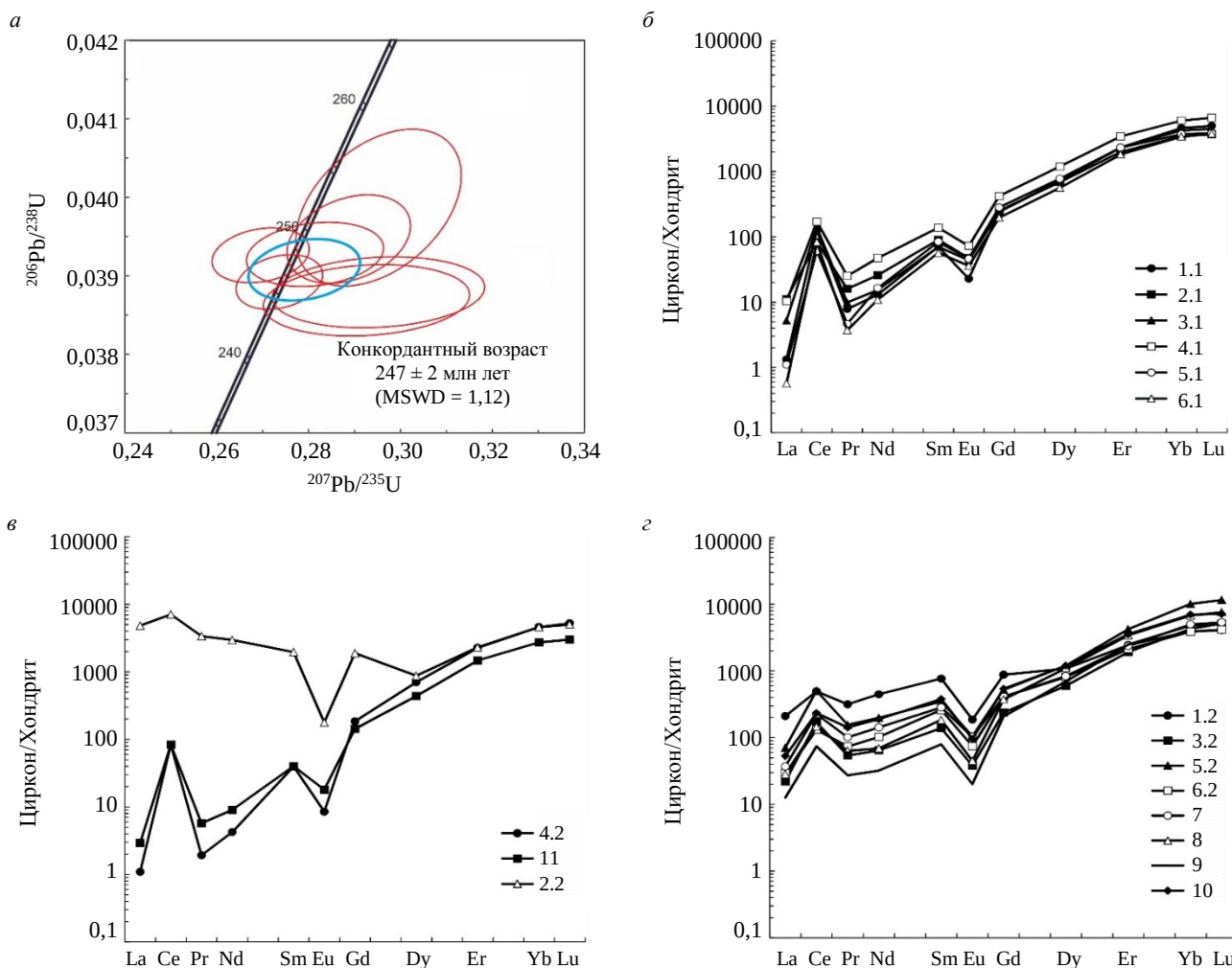
Рис.3. Диаграмма с конкордией (а) и спектры распределения REE (б-г), нормированные к хондриту CI, для циркона из гранитов второй фазы (обр. TH1-2)
