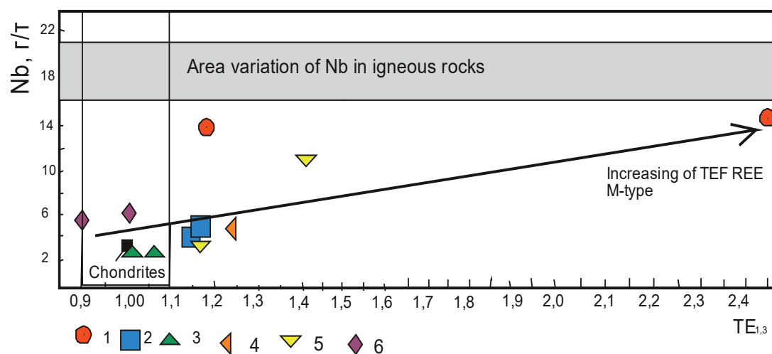
Рис. 8. Диаграмма \text{Nb}-\text{TE}_{1,3} для турмалина пегматитовых месторождений Горного Алтая. Серая область на диаграмме выделена на основании средних содержаний вольфрама в изверженных породах по [21]. Содержания вольфрама в хондритах по [22]. Условные обозначения – на рис. 2, б
