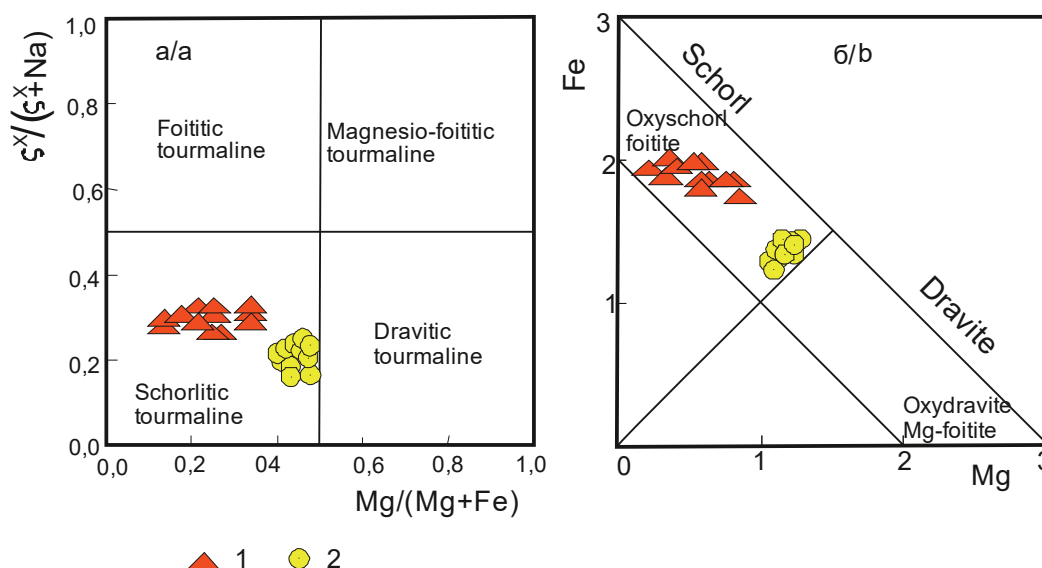
Рис. 1. Бинарные диаграммы \zeta^x/(\zeta^x+\text{Na}) –Mg/(Mg+Fe) (а) и Fe–Mg (б) в атомных количествах по [11] для турмалинов грейзеновых и пегматитовых месторождений Горного Алтая. Турмалин: 1 – грейзенов, 2 – пегматитов
