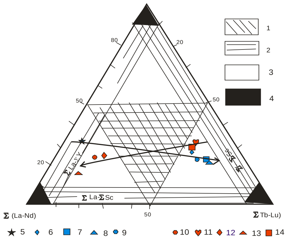
Рис. 5. Диаграмма \Sigma (La-Nd) - \Sigma (Sm-Ho) - \Sigma (Tb-Lu) составов РЗЭ в сталагмите
