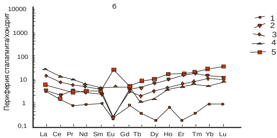
Рис. 4. Спайдер-диаграммы распределения РЗЭ в сталагмите: а- для центральной части, б- для периферии. Нормализация относительно хондрита по [21].
