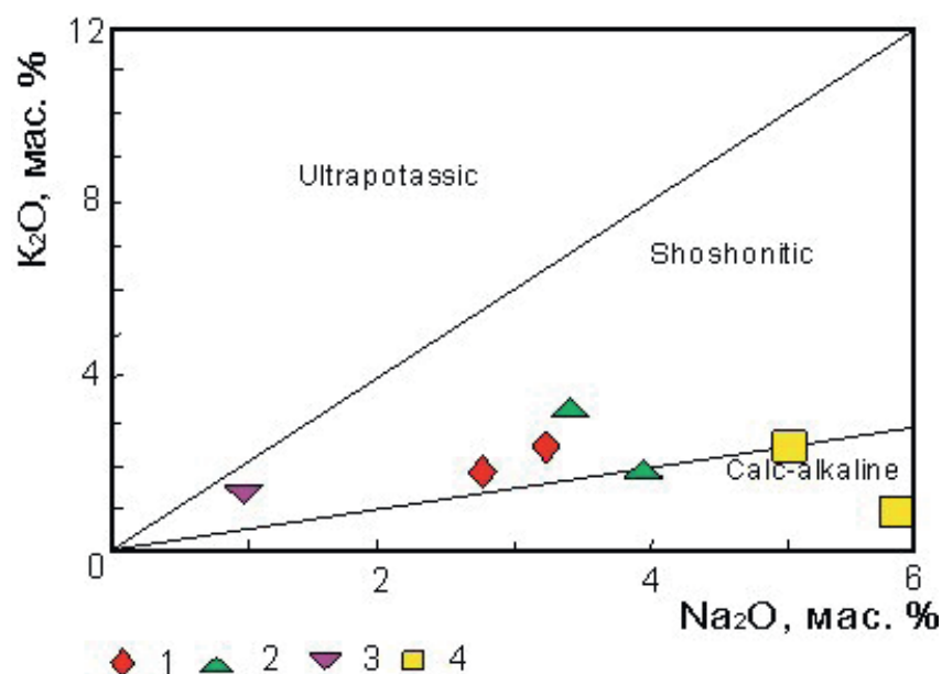
Рис. 4. Диаграмма K 2 O – Na 2 O по [Davidson et al., 2007] для интрузивных пород Тимофеевского штока. Серии пород: Calc-alkaline- известково-щелочная, Shoshonitic - шошонитовая, Ultrapotassic – ультрака- лиевая. Остальные условные на рис. 3.
