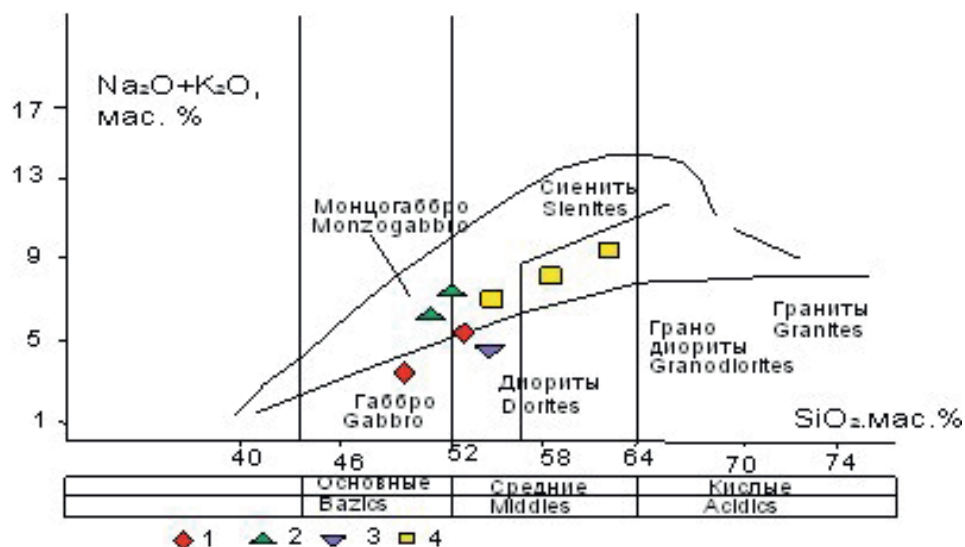
Рис. 3. Петрохимическая диаграмма диагностики горных пород в координатах SiO 2 – (Na 2 O+K 2 O) для пород Тимофеевского штока и вмещающих туфов.
