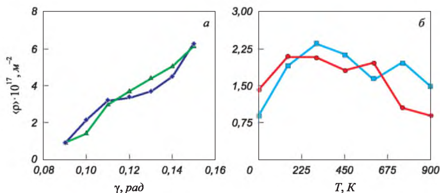
Рис. 3. Изменение средней плотности дислокаций \langle \rho \rangle при различных углах сдвига ( R = 16 Å) (а) при 0 К (▲) и 300 К (◆) и при различной температуре расчетной ячейки ( \gamma = 0,1 рад) (б), вычисленной на временном интервале 12,5 – 15,0 пс, и при радиусе основания цилиндрических пор 16 Å (●), 8 Å (■)
