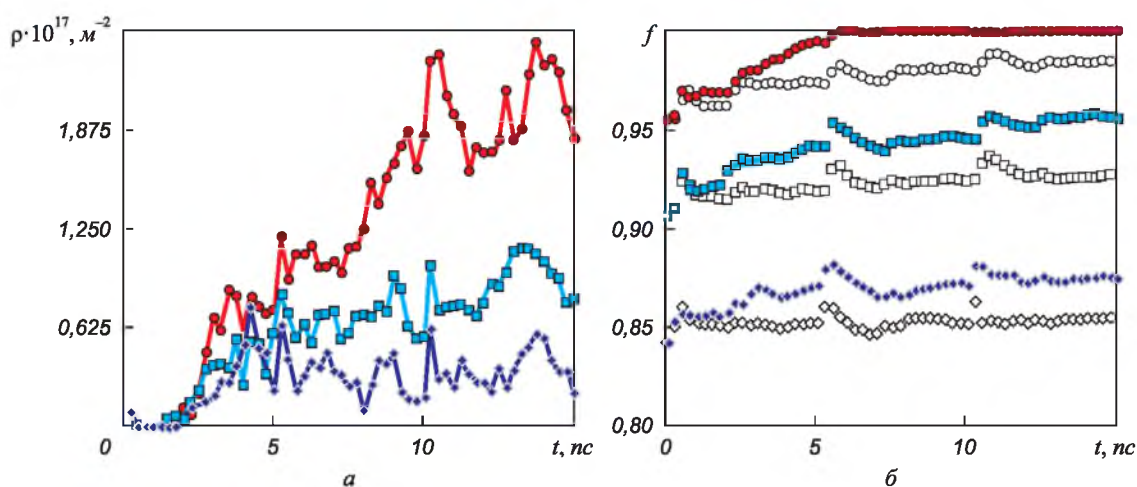
Рис. 5. Изменение плотности дислокаций \rho ( T = 300 К) (а) и объемной доли «фазы вещества» f (при T = 300 К (○, □, ◇) и T = 600 К (●, ■, ◆)) (б), при прохождении ударных волн, генерируемых в расчетной ячейке с интервалом 5 пс (угол сдвига \gamma = 0,07 рад): ● – 8 Å; ■ – 12 Å; ◆ – 16 Å
