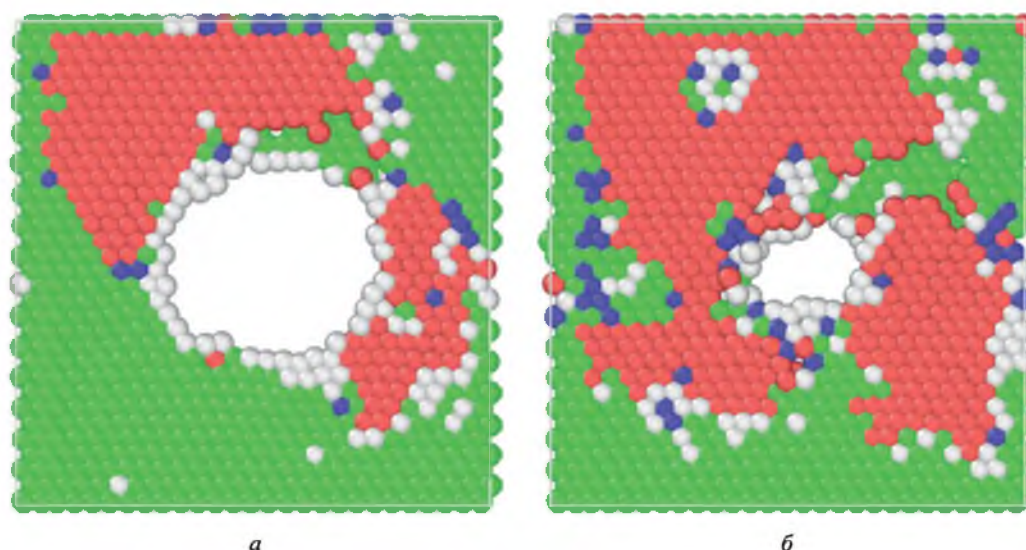
Рис. 4. Фрагмент плоскости (111) расчетной ячейки, содержащей пору с радиусом основания 16 Å (а) и 8 Å (б), через 5 пс после генерации ударной волны при T = 300 К. Цветовая визуализация соответствует распределению локального окружения атомов: ГЦК (зеленый), ГПУ (красный), ОЦК (синий), не определено (белый)
