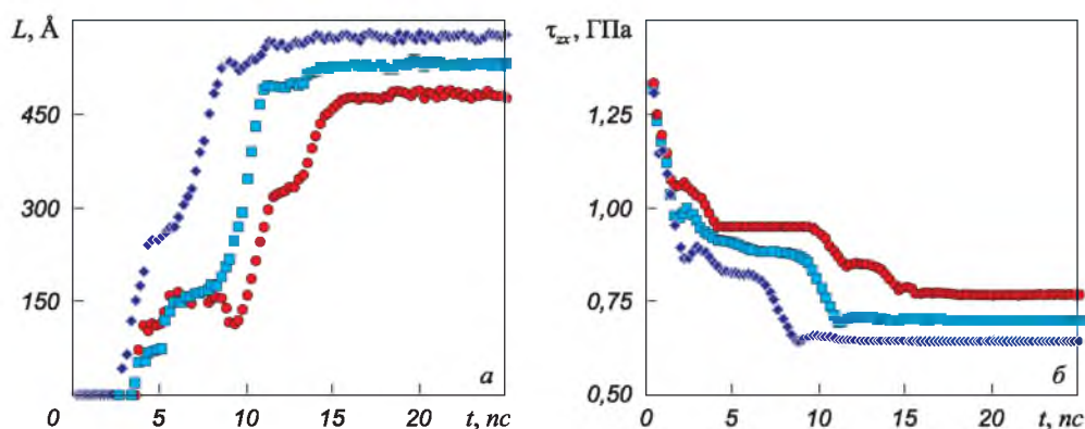
Рис. 2. Изменение суммарной длины L дислокационных петель (а) и касательных напряжений в расчетной ячейке (б) в процессе моделирования при радиусах R основания цилиндрических пор 8 Å (●), 12 Å (■) и 16 Å (◆). Угол сдвига \gamma = 0,1 рад
