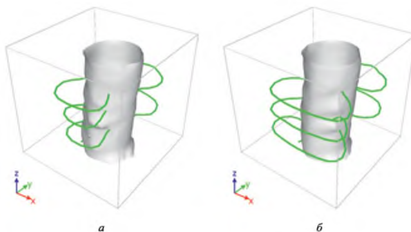
Рис. 1. Визуализация развития дислокационной структуры в процессе моделирования через 1500 (а) и 5000 (б) шагов вычислений. Угол сдвига \gamma = 0,1 рад
