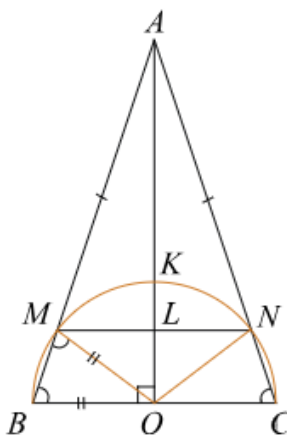
Рис. 1. Сечение комбинации конуса и полусферы
