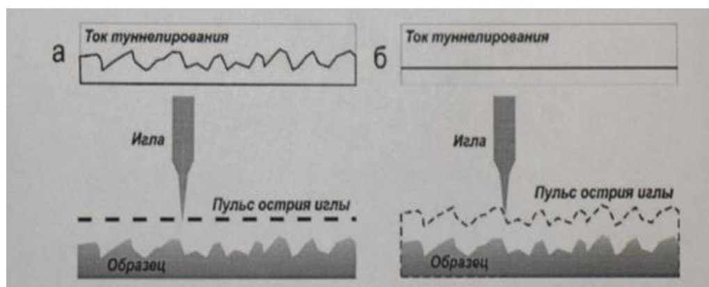
Рис. 1. Схема действия сканирующего туннельного микроскопа:
