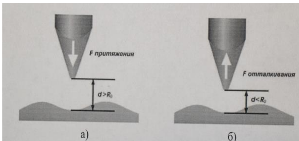
Рис. 2. Схема действия атомно-силового микроскопа: а) бесконтактный режим; регистрация сил притяжения; б) контактный режим; регистрация сил отталкивания.
