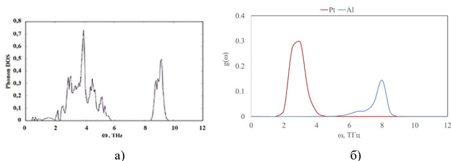
Рис.1. Плотность фононных состояний: а) рассчитанная средствами LAMMPS, который включает необходимые для этих целей процедуры, базирующиеся на преобразовании Фурье автокорреляционных функций перемещений атомов от времени [20], б) рассчитанная в рамках предложенного алгоритма при температуре 450 K
