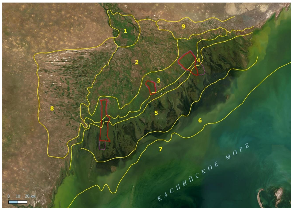
Рис. 1. Современное расположение участков Астраханского государственного заповедника в соответствии со схемой деления дельтовой области реки Волги по Е.Ф. Белевич: 1 – верхняя зона дельты; 2 – средняя зона дельты; 3 – нижняя зона дельты; 4 – култушная зона дельты; 5 – островная зона авандельты; 6 – зона открытой авандельты; 7 – зона морского подхода к авандельте; 8 – западный ильменно-бугровой район; 9 – восточный ильменно-бугровой район
