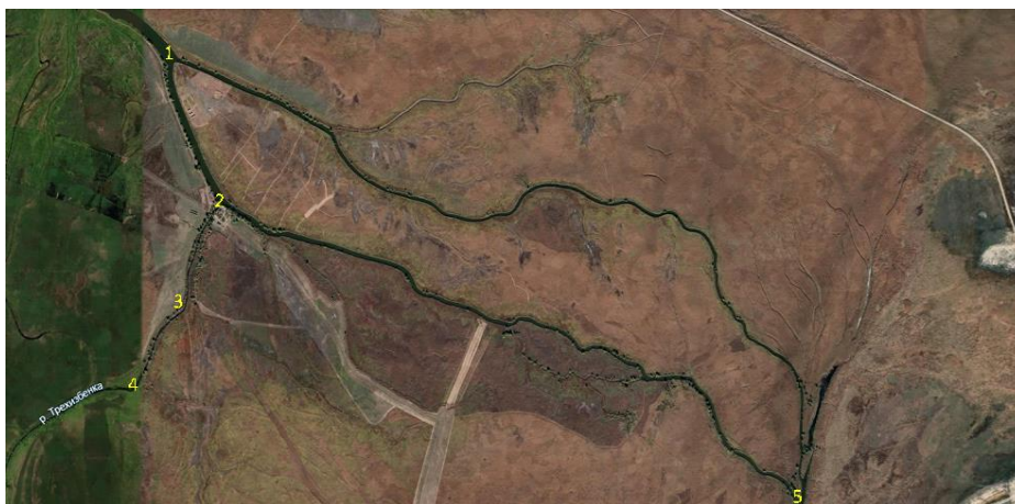
Рис. 2 «Карта-схема расположения точек для отбора проб». 1 – «До фермы», 2 – «Кордон», 3 – «Мелководье», 4 – «Яма», 5 – «После фермы»
