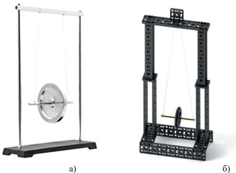
Рисунок 1. а) Маятник Максвелла; б) Маятник Максвелла из робототехнического набора Pimnara.
