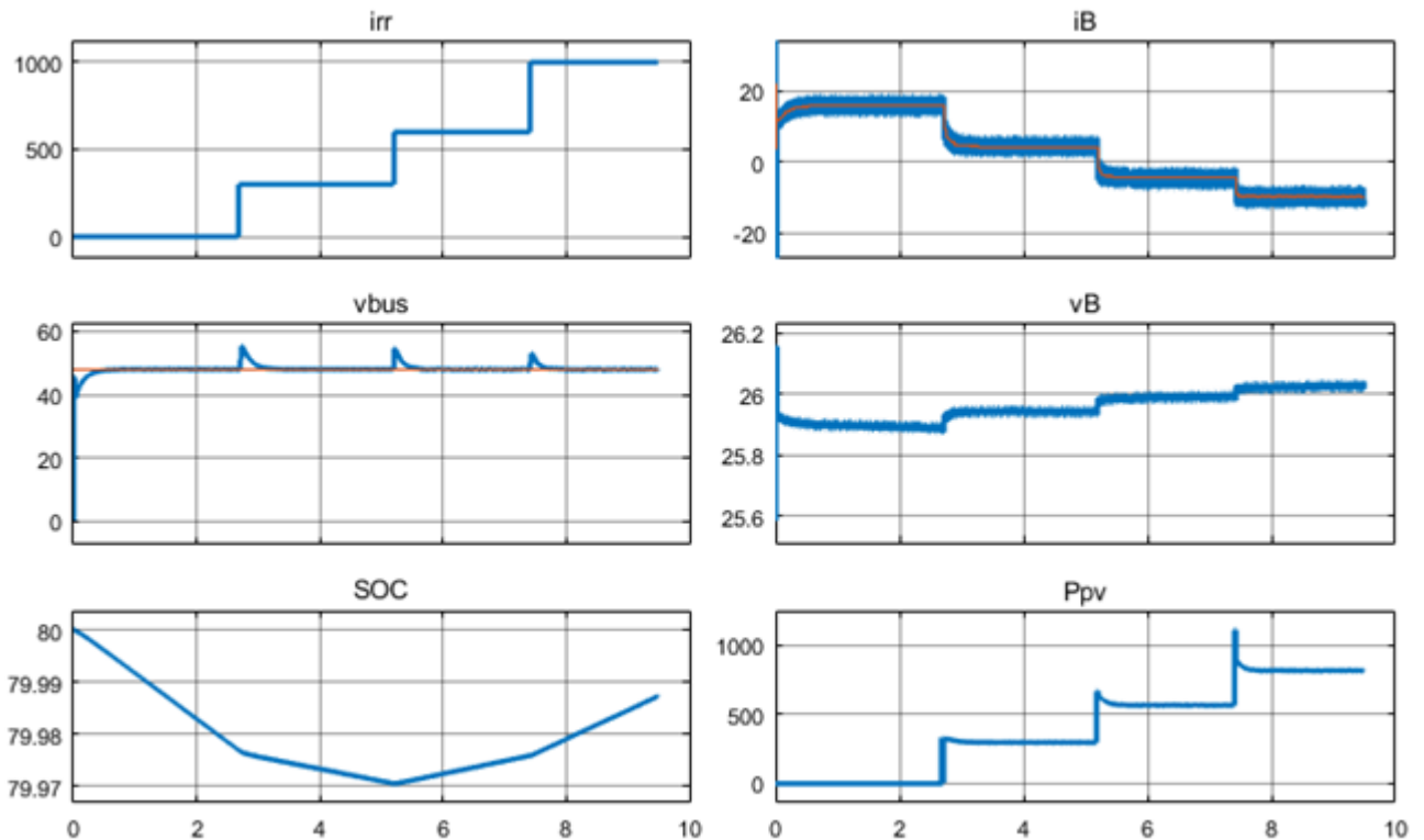
Рис. 1. Осциллограммы интенсивности излучения irr , напряжения шины постоянного тока v_{bus} , степени заряда аккумуляторной батареи SOC, тока аккумуляторной батареи i_B , напряжения аккумуляторной батареи v_B , мощности солнечной батареи P_{pv}
