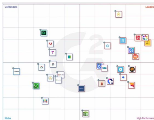
Рисунок 1. Authoring tools
