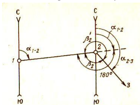
Рис. 2. Схема определения горизонтального угла
