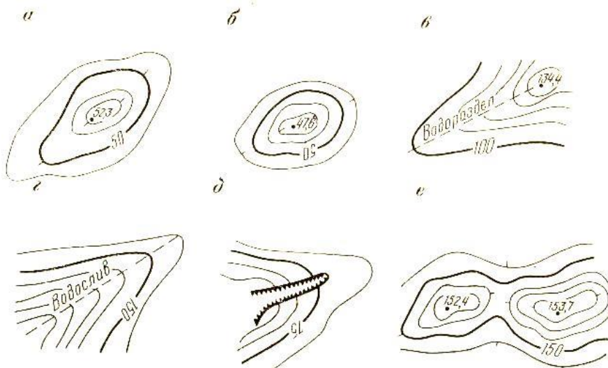
Рис. 3. Схема изображения основных форм рельефа горизонталями
