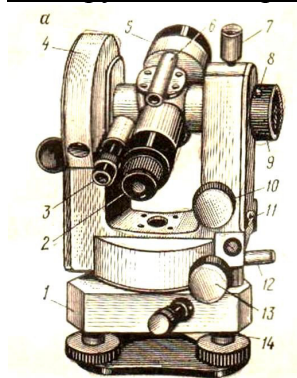
Рис. 1 Теодолит Т30
