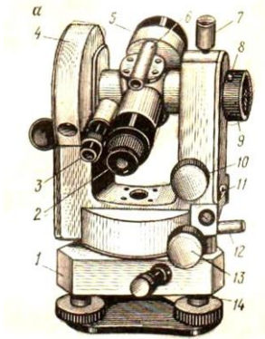
Рис. 1 Теодолит Т30
